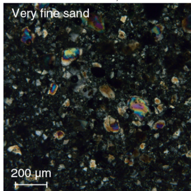
U1518E-12F-3, 25 cm
