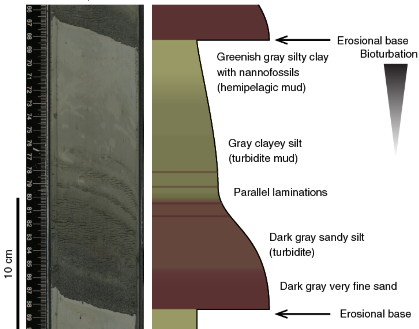
U1518E-2H-3, 108 cm
