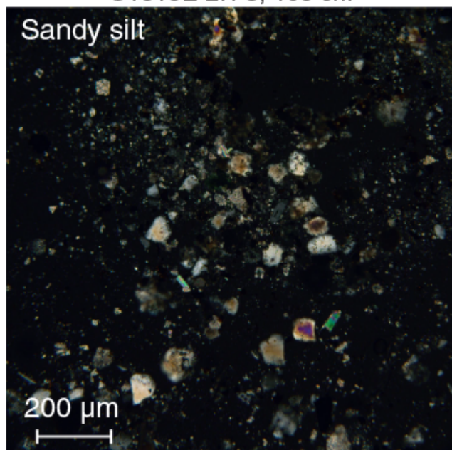
U1518E-2H-3, 108 cm
